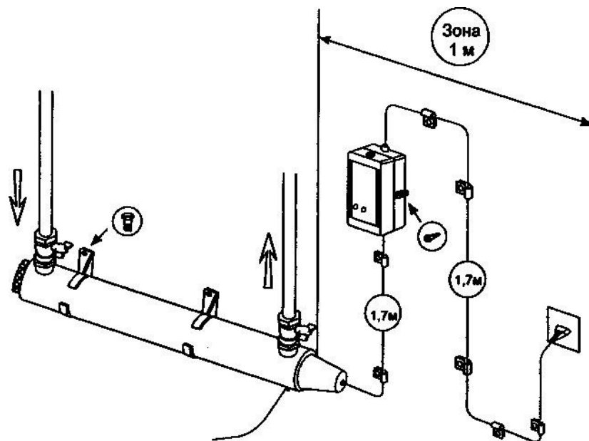
Пример монтажа установки в горизонтальном положении
